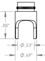
S2L 2-Leg Cutter Ø1/2" (Ø12mm)
