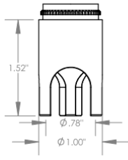
S3L 3-Leg Cutter \phi 3/4" ( \phi 19 mm)
