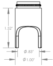
S2L 2-Leg Cutter \phi 3/4" ( \phi 19 mm)
