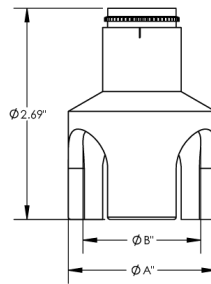
S3L 3-Leg
